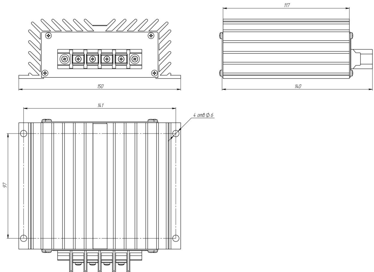
Рисунок 2. ПН1-50Г общий вид
