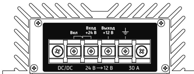
Рисунок 3 Передняя панель ПН1-50Г
